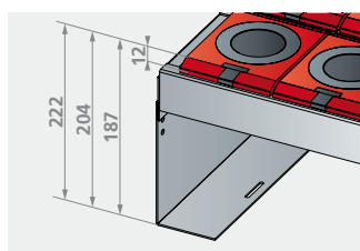
Para alturas de almacenamiento de 187-222 mm (27 E y 36 E)
