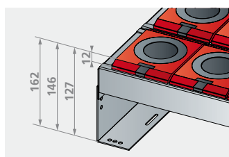
Para alturas de almacenamiento de 127-162 mm (27 E y 36 E)
