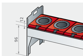
Para alturas de almacenamiento de 96/135 mm (27 E y 36 E)
